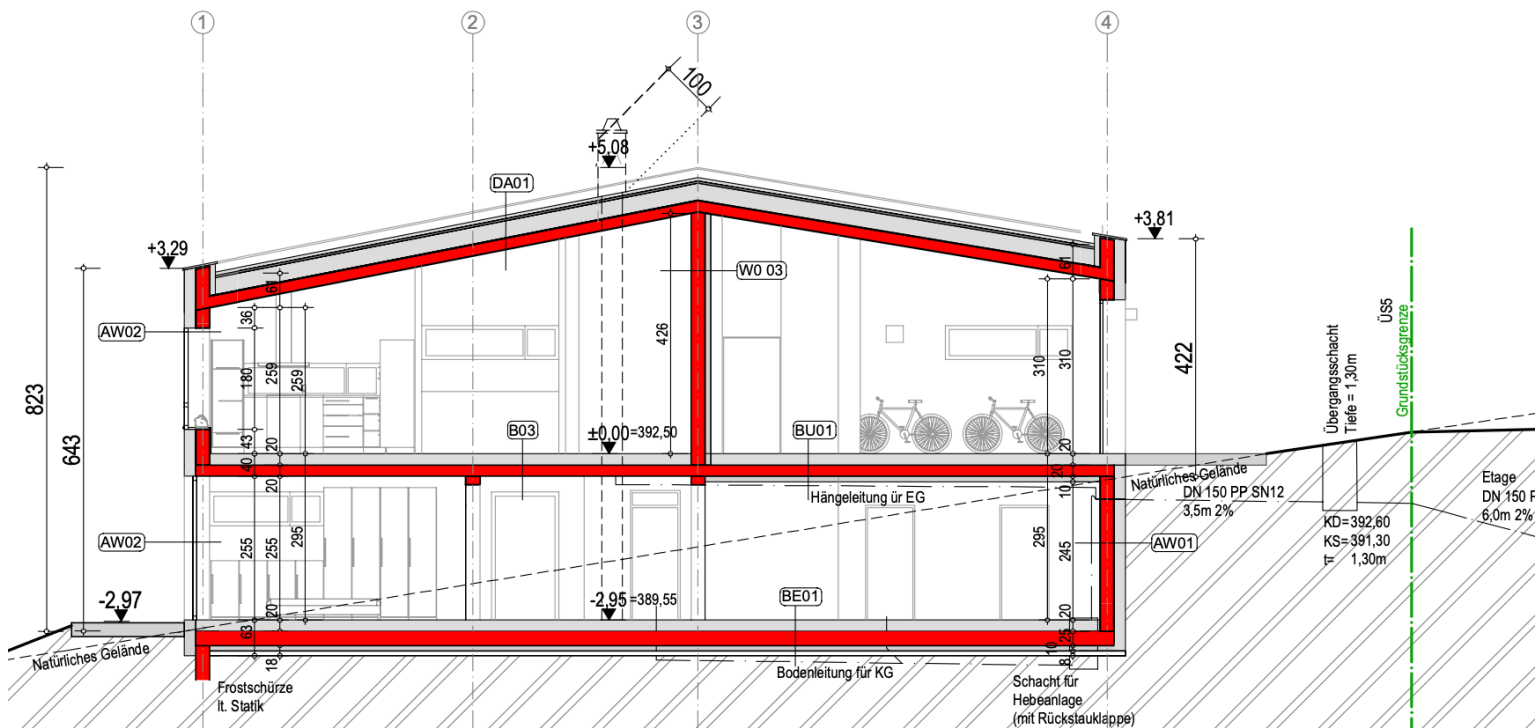
SCHNITT A 1:100
