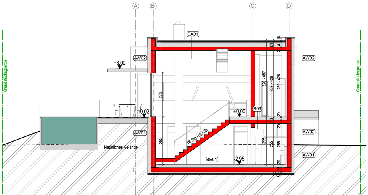
SCHNITT A 1:100
